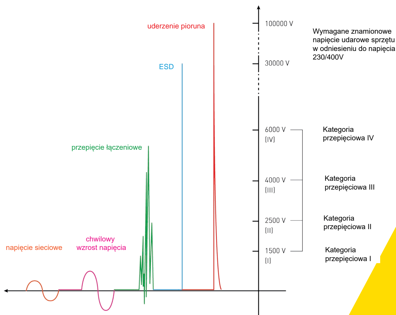
Rys. 2: Typy przebiegów i ich amplitudy
