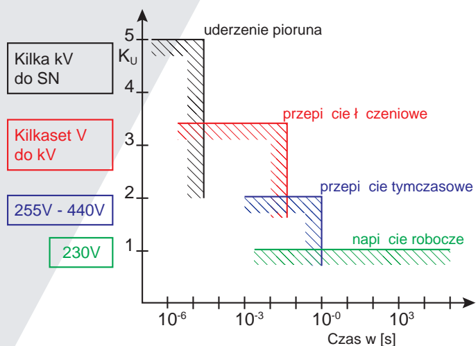
Rys. 1: Poziomy napięcia w systemie zasilania energia
