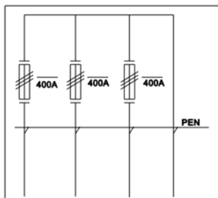
Układ sieci TN-C
