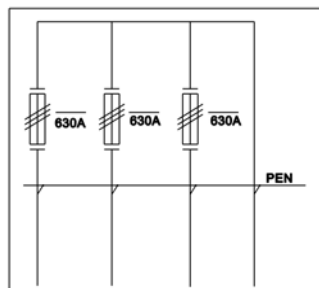
Układ sieci TN-C
