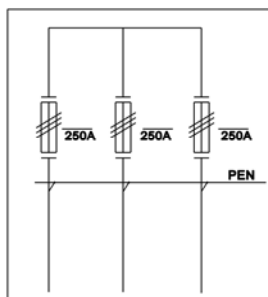
Układ sieci TN-C
