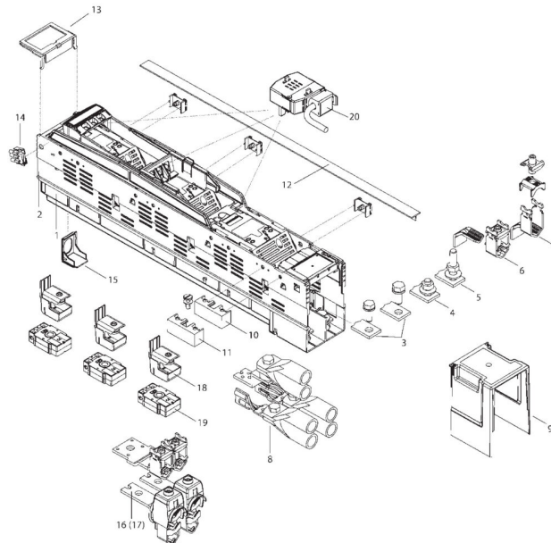
Rozłączniki bezpiecznikowe listwowe typu SL1-3X3, SL2-3X3, SL3-3X3 Osprzęt do aparatów na system szyn zbiorczych o rozstawie 185 mm, rozłączanych 3-biegunowo
